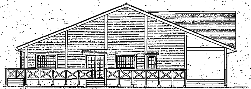
北立面図
