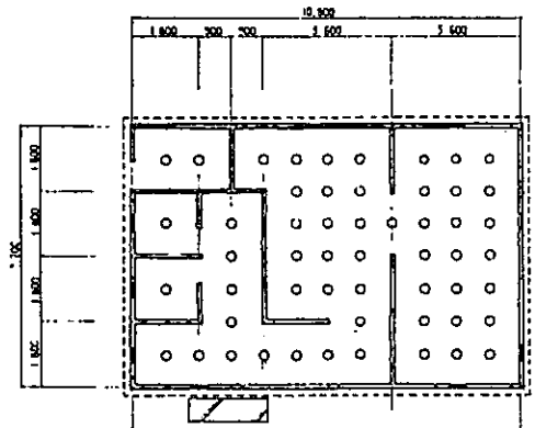
小館 1/100
