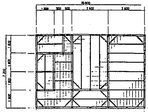
本館 1/100
