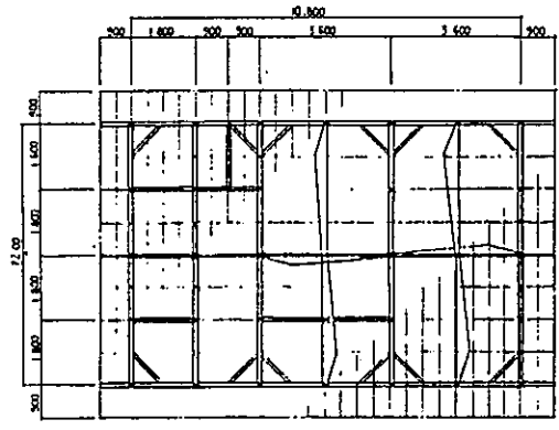
小館 1/100
